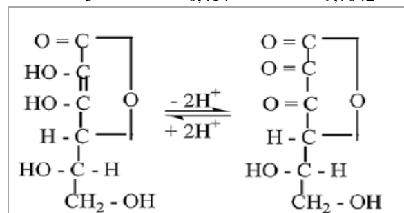
Asam -L-askorbat Asam -L-dehidroaskorbat
